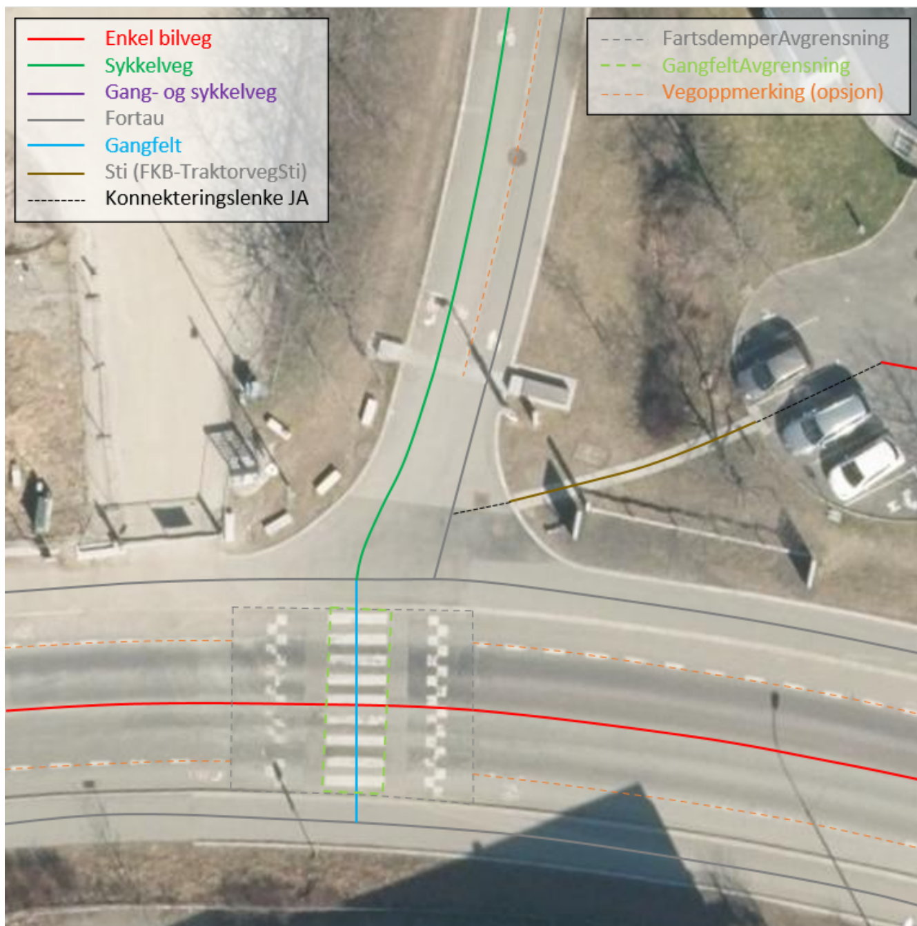
Figur 4. Eksemplet viser hvordan veglenkene i Elveg skal henge sammen. Det presiseres at ved parallelle lenker forlenges hver lenke (her sykkelveg og fortau) mot nærmest tilstøtende veglenke (her fortau).
