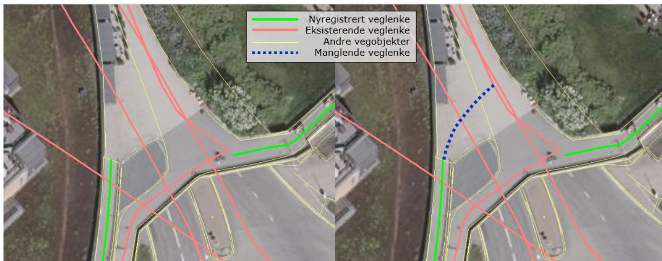
Figur 14. Et eksempel på kortere veglenke (>2m) som danner topologi mellom to gang- og sykkelveger.
