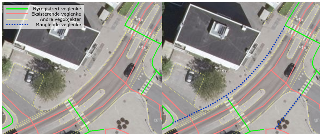
Figur 19. Eksempelet viser en veglenke som går over en litt lengre strekning men som samtidig har nyregistrerte veglenker i begge ender (med typeveg fortau). Derfor skal denne typen veglenker registreres fotogrammetrisk. Veglenke skal registreres med typeveg fortau som knyttes sammen med nyregistrerte fortau i både nordøst og sørvest. Eksempelet viser også en manglende veglenke fra gangfelt til eksisterende gang- og sykkelveg, som kan beskrives som en kortere veglenke som skal registreres fotogrammetrisk, se kapittel "Korte (>2m), naturlige forbindelser for gående og syklende".
