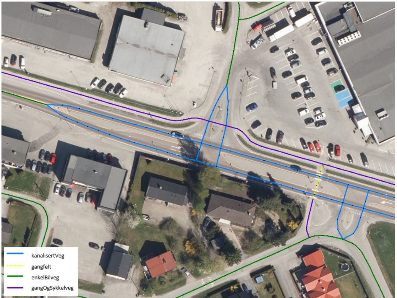
Figur 2. Figuren viser registrering av flere ulike typer veg i et fullkanalisert T-kryss med svingefelt. I de aller fleste tilfeller vil topologien i slike kryss være etablert og skal da ikke endres ved fotogrammetrisk registrering. Fotogrammetrisk registrering vil i hovedsak gå ut på forbedring av geometri der kriteriene for dette er tilstede.
