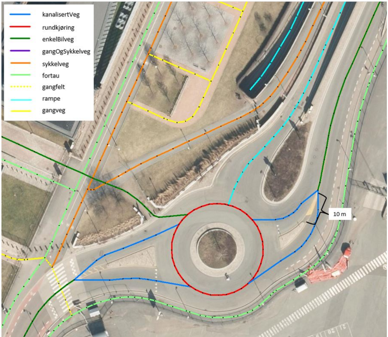
Figur 3. Figuren viser registrering av flere ulike typer veg
