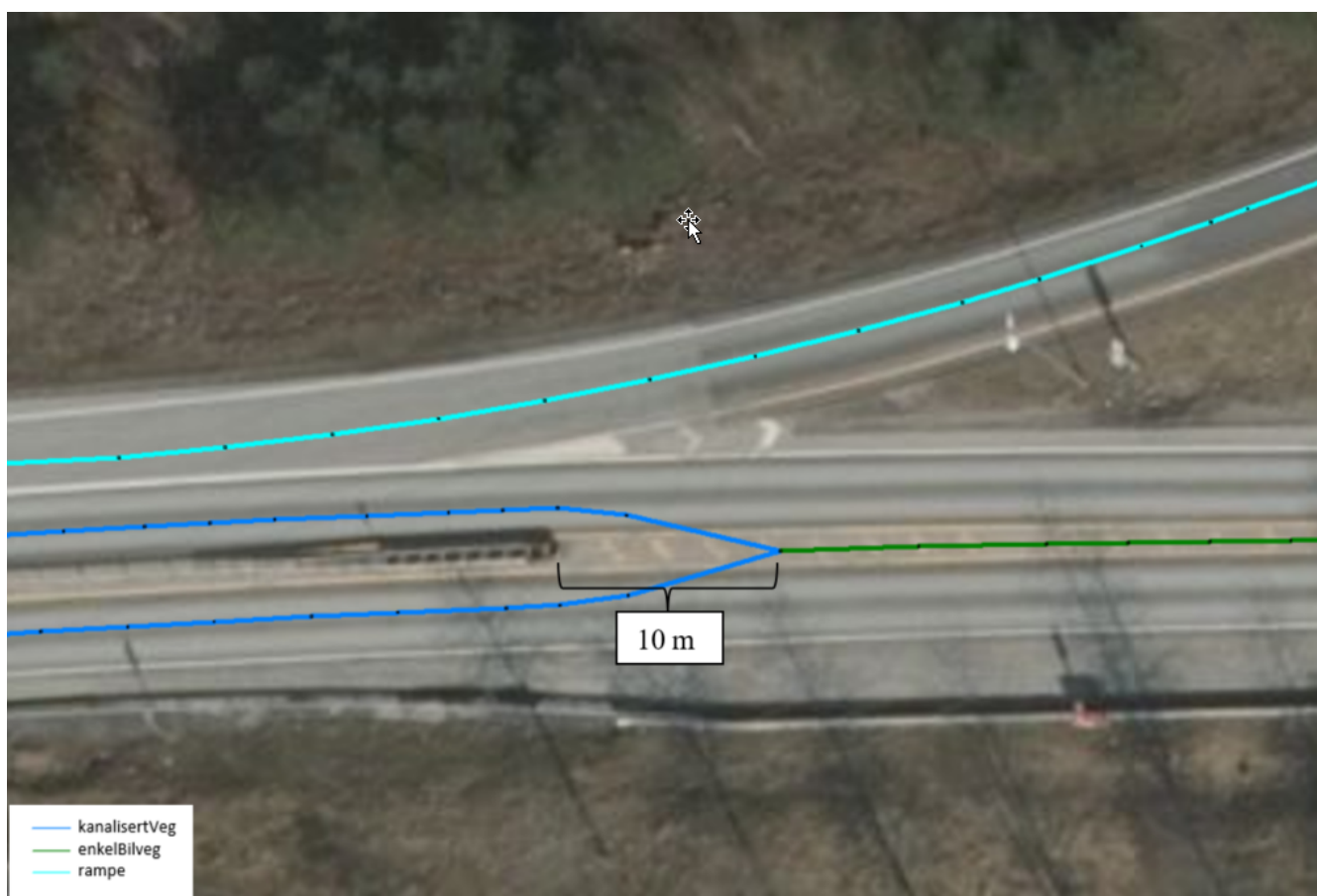
Figur 6. Start- og sluttunkt for kanalisert veg settes normalt 10 meter før- og etter fysisk hinder
