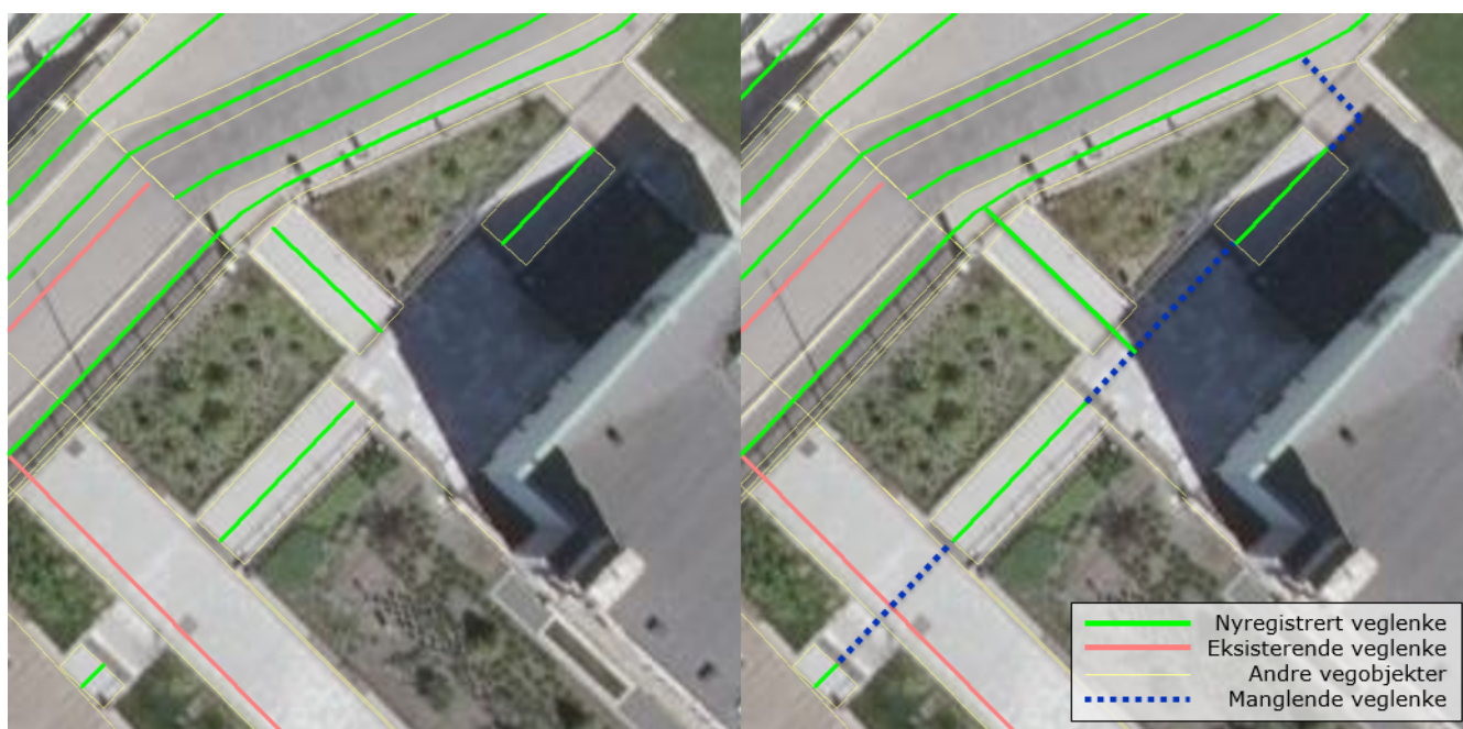
Figur 15. Når avstanden er kortere enn 2m skal trapp forlenges mot nærmeste veglenke. Når avstanden er over 2m skal egen veglenke registreres, fortrinnsvis med typeveg gangveg mellom trapper og/eller mot tilgrensende veglenker for gående (se bildeeksempel til høyre).
