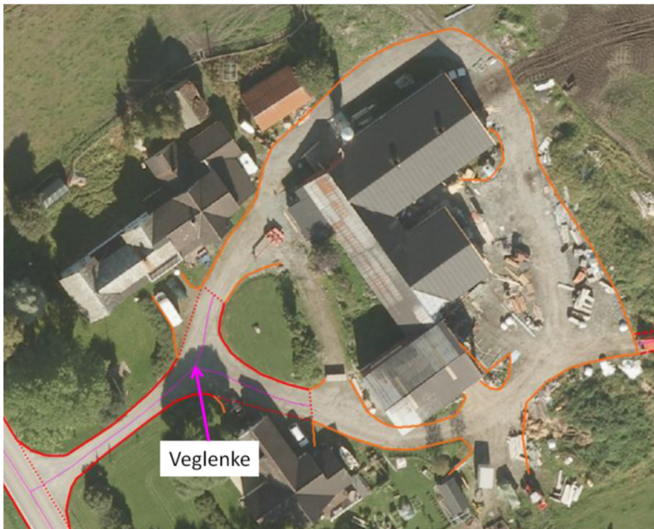
Figur 24. Eksempel på riktig avslutning av veglenke (og vegflate i FKB-Veg) på gårds plass. Det skal ikke registreres veglenke rundt driftsbygningen i dette tilfellet. NB! Bildet viser overfullstendighet av AnnetVegarealAvgrensning rundt rundt driftsbygningen
