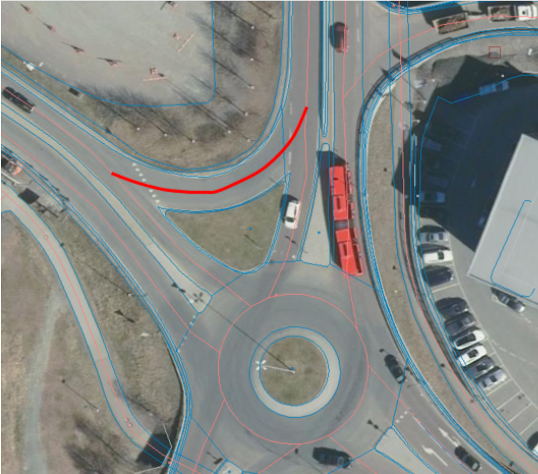
Figur 22. Eksemplet viser registrering av veglenke med typeveg kanalisert veg for svingefelt.
