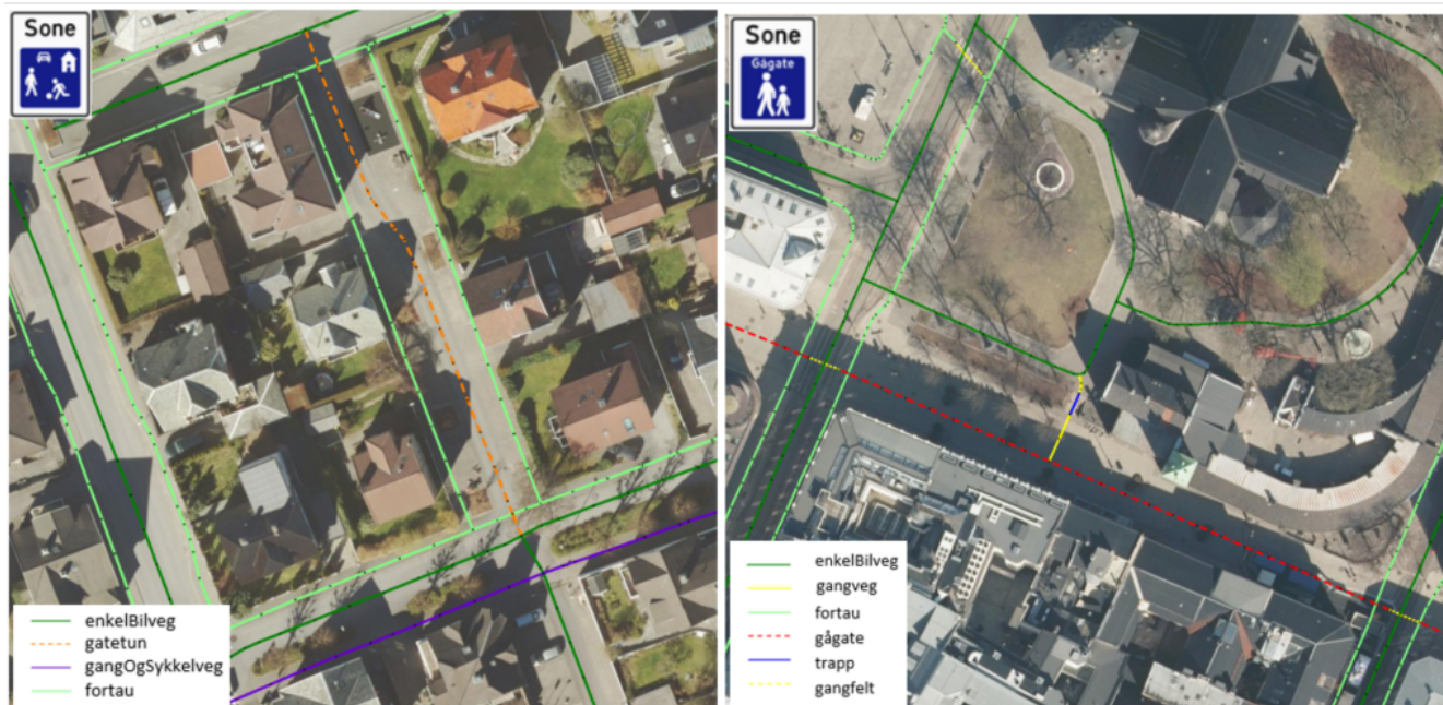
Figur 5. Venstre skisse viser eksempel på gattetun. Høyre skisse viser gågate
