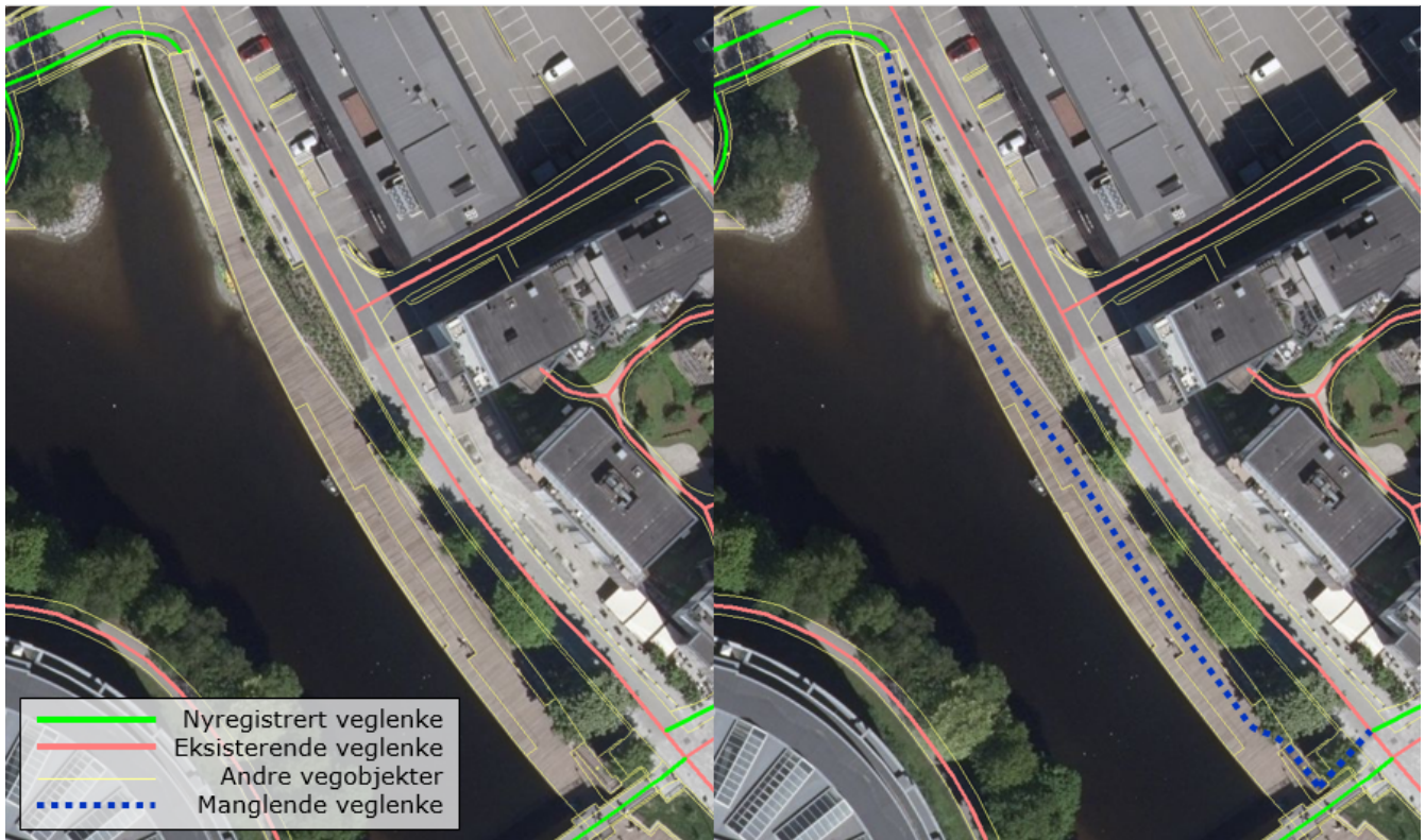
Figur 16. Eksempelet viser en veglenke som kan registreres (med typeveg gangveg) etter manus. Denne skal knyttes sammen mot fortau i nord og mot fortau (manglende veglenke for trapp og veglenke videre fra trapp mot fortau vises også i blått i bildet) i sørøst.
