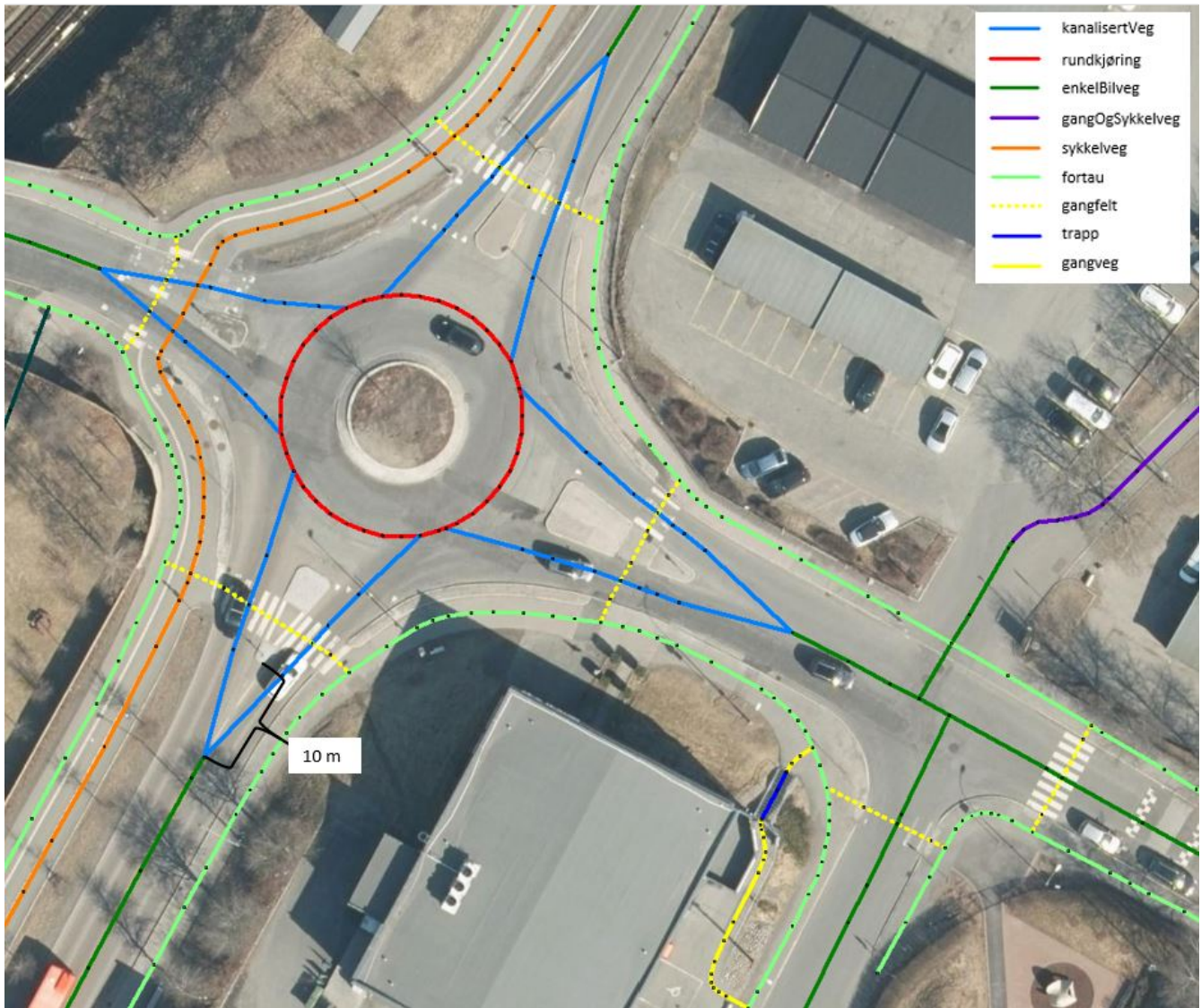
Figur 1. Figuren viser eksempel på registrering av flere ulike typer veg. Rundkjøring registreres i senter av sirkulasjonsarealet uavhengig av antall kjørefelt
