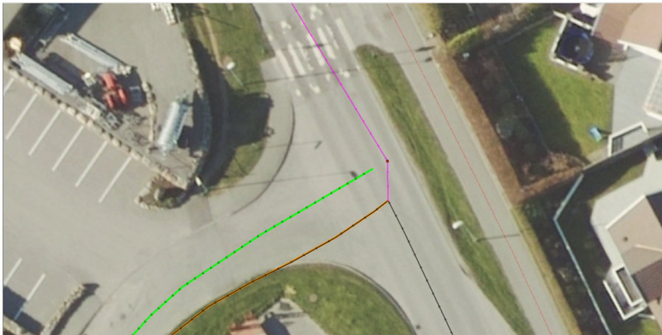
Figur 23. Eksempel på riktig avslutning av veglenke mot eksisterende geometri. Markert lenke (rosa) er eksisterende lenke som er innenfor kvalitetskrav ( \pm 2m ). Nykonstruert lenke (grønn) skal da konstrueres til midt av vegen slik bildet viser. Da er den nykonstruerte lenka helt riktig og den eksisterende lenka med litt dårlig geometri, men ikke så dårlig at den skal nykonstrueres, vil bli riktig tilpasset ny geometri ved innlegging i NVDB. Oransje lenke er kodet med Endret type S og skal slettes
