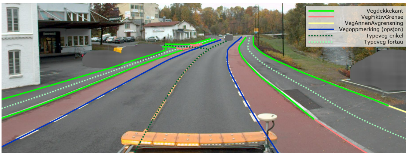
Figur 21. Eksempel på registrering av sykkelfelt i vegbanen. Sykkelfelt har ingen egen veglenke i FKB 5.0. Den inngår i vegflaten og avgrensningen av sykkelfeltet registreres med objekttypen vegoppmerking (opsjon). For beskrivelse av objekttyper og typeveg, se bilde.
