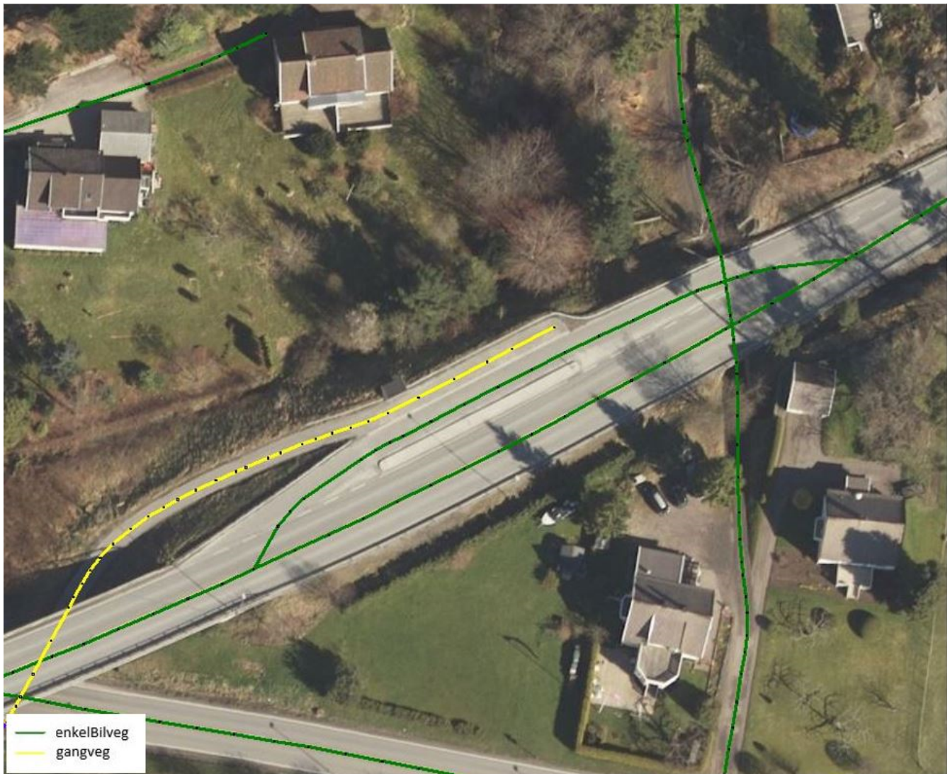
Figur 9. Eksempel på start/slutt nyregistrert gangveg ved busslomme. Fysisk adskilt trafikklomme registrert som enkel bilveg. Dette er et eksempel på "lovlig løs ende" i nettverket for gående.
